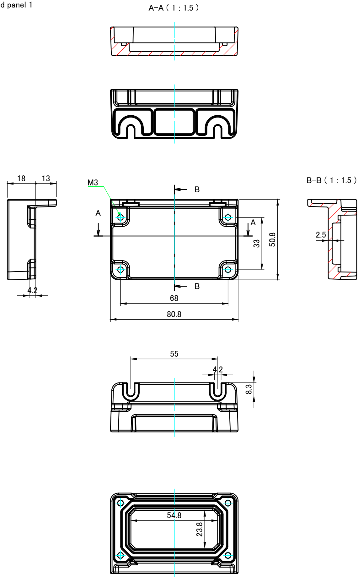
フランジ付側板1 Flanged end panel 1
